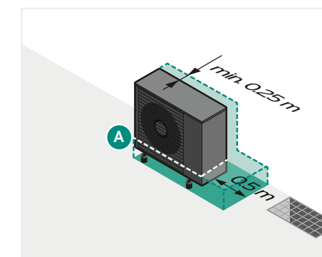
aroTHERM plus/8 nach Aktivierung der Funktion
