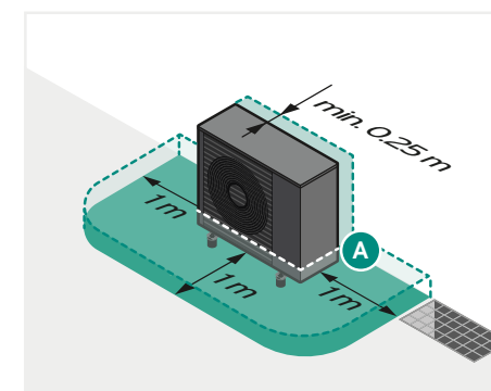
aroTHERM plus/8 vor Aktivierung der Funktion
