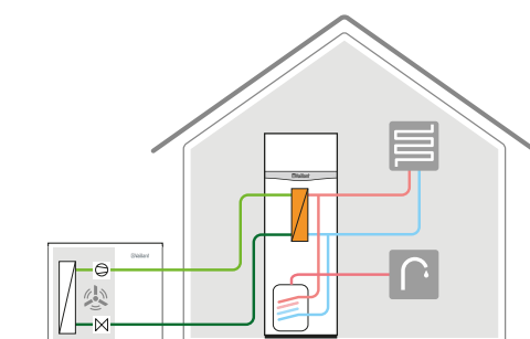
split-System: Verflüssiger in der Inneneinheit
