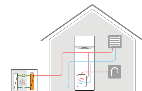
Monoblock-System: alle Wärmepumpen- Komponenten in der Außeneinheit
