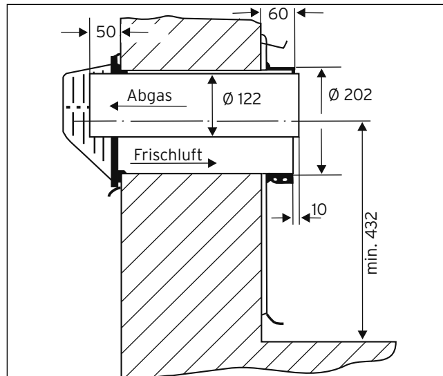
5.9 Mauerquerschnitt mit normaler Windschutzeinrichtung
