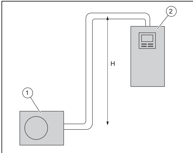
1 Außeneinheit 2 Inneneinheit
